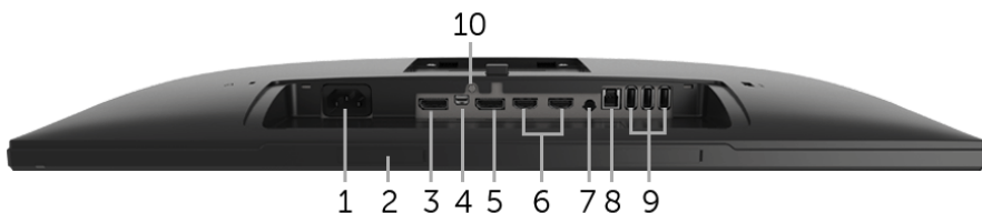
Вид снизу без стойки монитора
